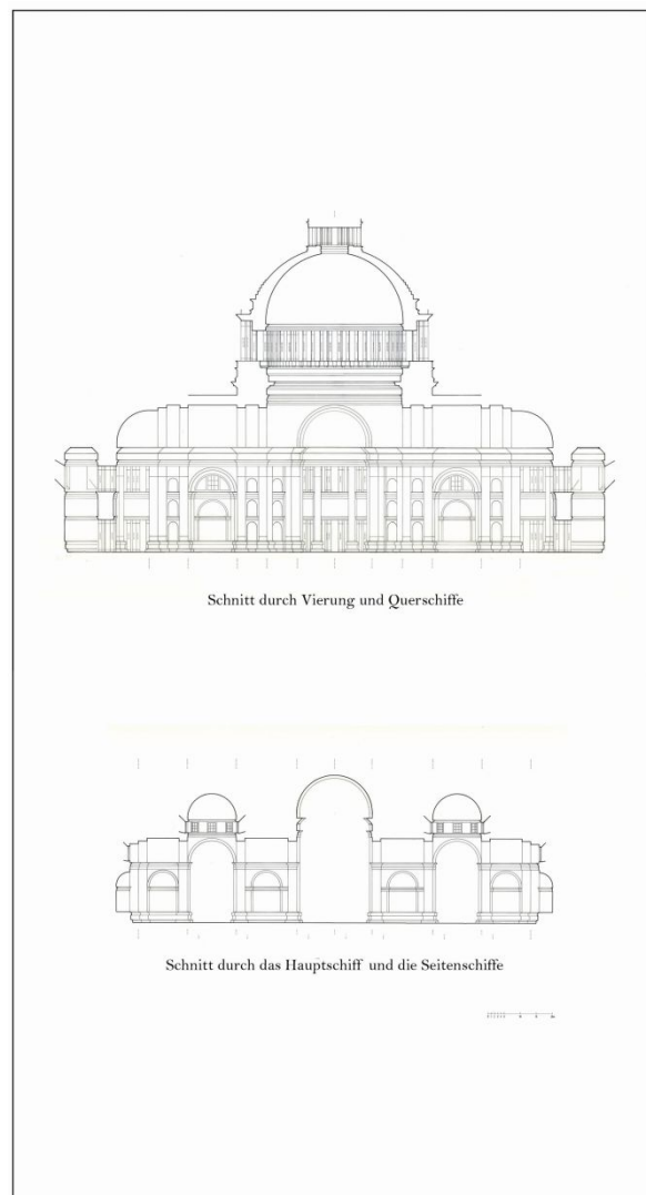
Schnitte
