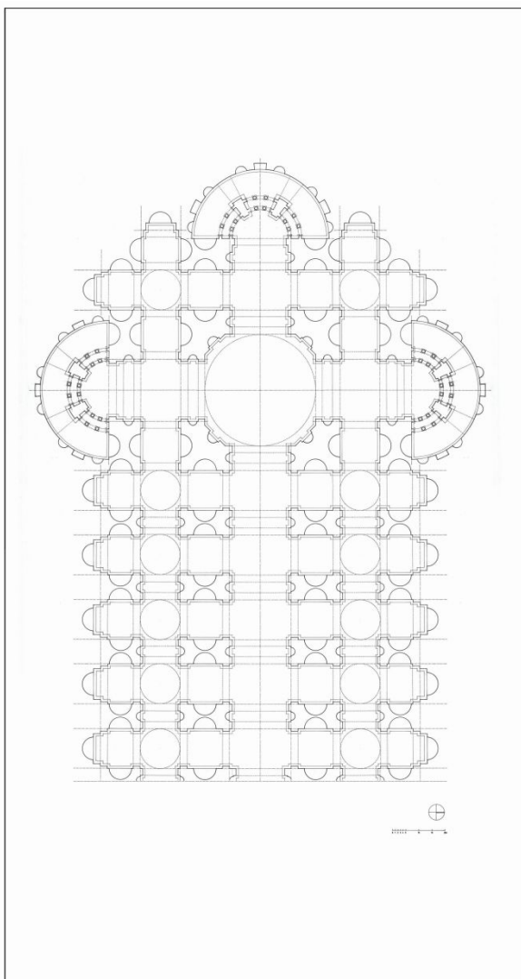
Grundriss
